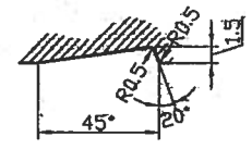
A-A SECTION SCALE=2:1
