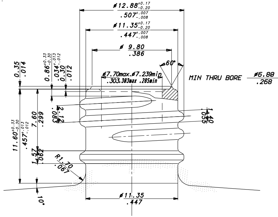
PART. IMBOCCATURA SCALA 5 : 1
